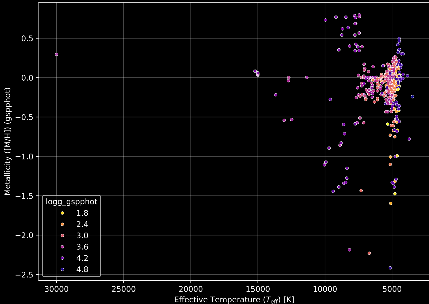
APOGEE DR17 Field: [150-04] Stellar Population Parameters (n= 483)
